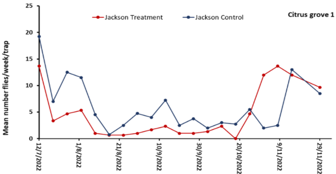
Διάγραμμα 1. Συλλήψεις ατόμων της μύγας της Μεσογείου σε παγίδες τύπου Jackson στα δύο τμήματα του αγρού 1 (πορτοκαλιάς ποικιλίας Washington Navel) (κόκκινη γραμμή: τμήμα αγρού με παγίδες, μπλε γραμμή: μάρτυρας).
